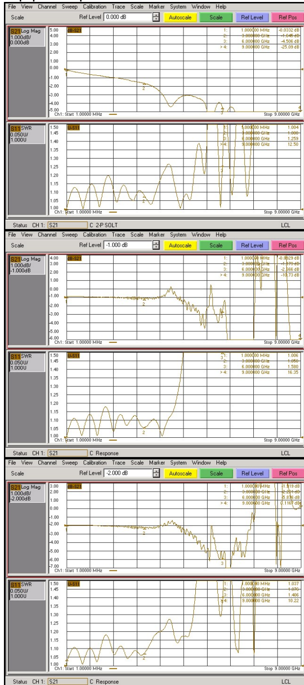
Графики для АЧХ - Log Mag, при аттенуаторе, установленном на 0 дБ, и для КСВ – SWR
