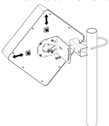
Рисунок 3 – X-поляризация
