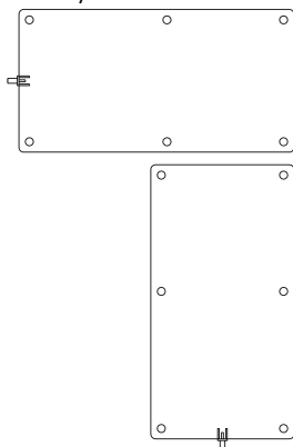
Рисунок 1 – Установка антенн в горизонтальной и вертикальной поляризациях
